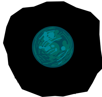
Pluto
