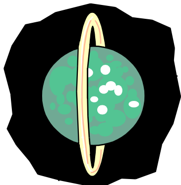
Uranus
